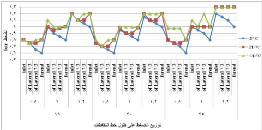
شكل (٦) يوضح تأثير تصميمات الأنظمة المستخدمة على توزيع الضغط داخل شبكة الري لنقاط (Pressure Compensating).
