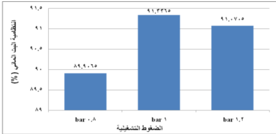
شكل (١١): تأثير الضغوط التشغيلية على انتظامية البث المائي .
