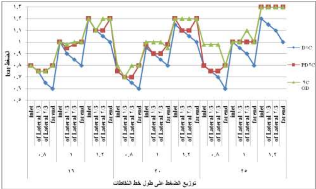
شكل (٥) يوضح تأثير تصميمات الأنظمة المستخدمة على توزيع الضغط داخل شبكة الري لنقاط (Turbulent).
