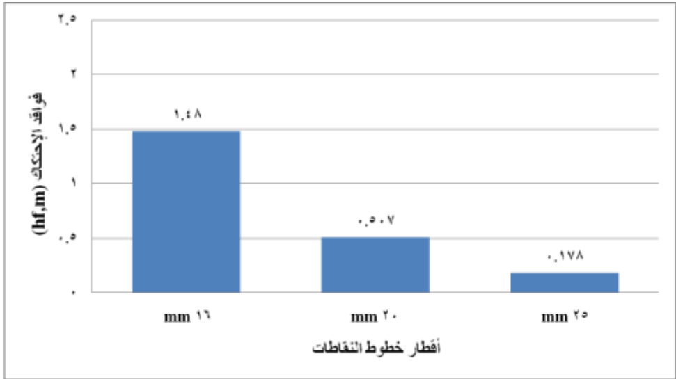
شكل (١٠): تأثير أقطار خطوط النقاطات على فاقد الاحتكاك .
