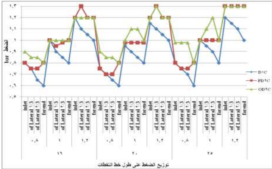
شكل (٧) يوضح تأثير تصميمات الأنظمة المستخدمة على توزيع الضغط داخل شبكة الري
