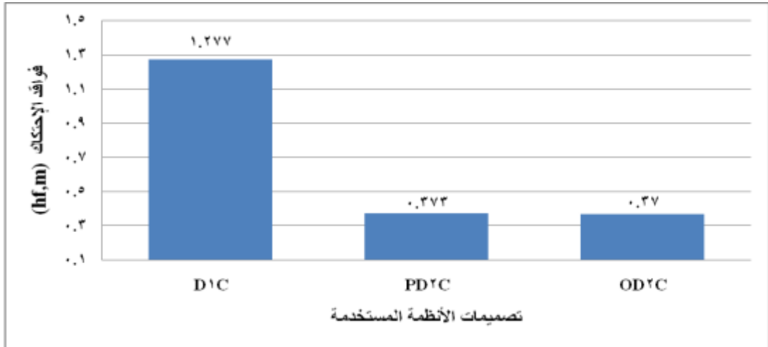
شكل (٤): تأثير تصميمات الأنظمة المستخدمة على فواقد الإحتكاك .
